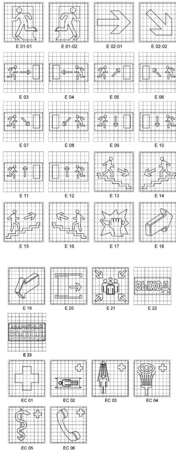
Рисунок П.5* - Эвакуационные знаки и знаки медицинского и санитарного назначения
