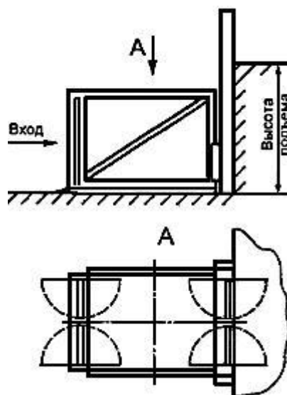
Рисунок 2 - Подъемная платформа без ограждения шахты
