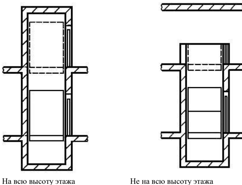
Рисунок 1 - Подъемная платформа в огражденной шахте
