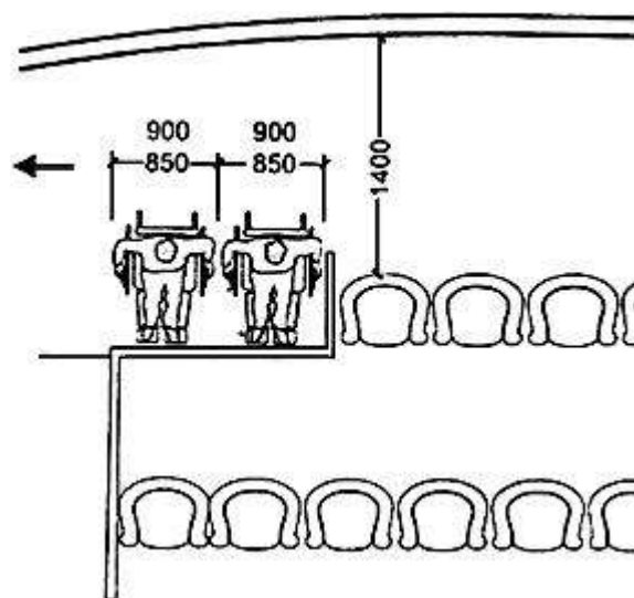
Рис 6.7. Места для инвалидов в зрительных залах
