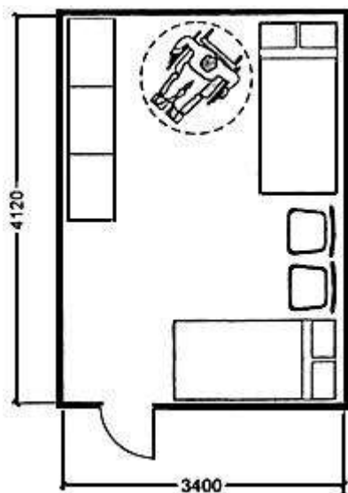
Рис 8.3. Гостиничные номера для инвалидов при вокзале Схема оборудования номеров для инвалидов в гостинице при вокзале
