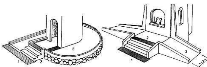
Устройство доступного для инвалидов подхода к местам поклонения
