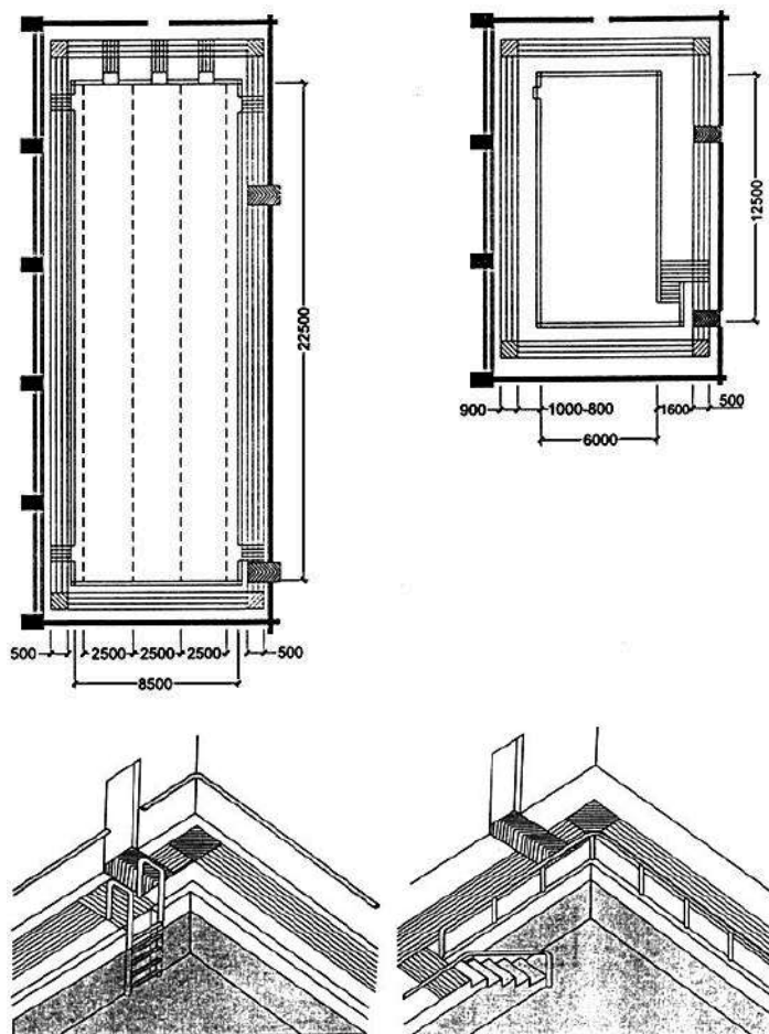
Рис 5.3. Плавательный бассейн Оборудование ванн бассейнов, посещаемых детьми-инвалидами
