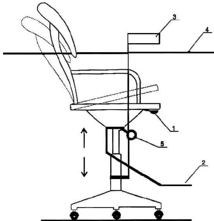
Рис. 13. Трансформируемый рабочий стол для инвалида
