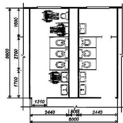
Цеховая уборная с кабиной для инвалидов
