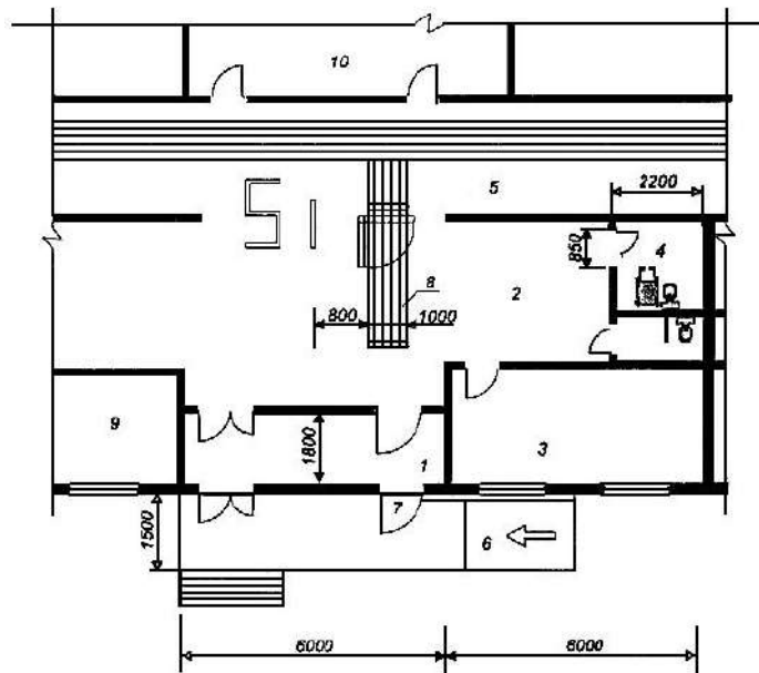
Рис. 2. Встроенный контрольно-пропускной пункт
