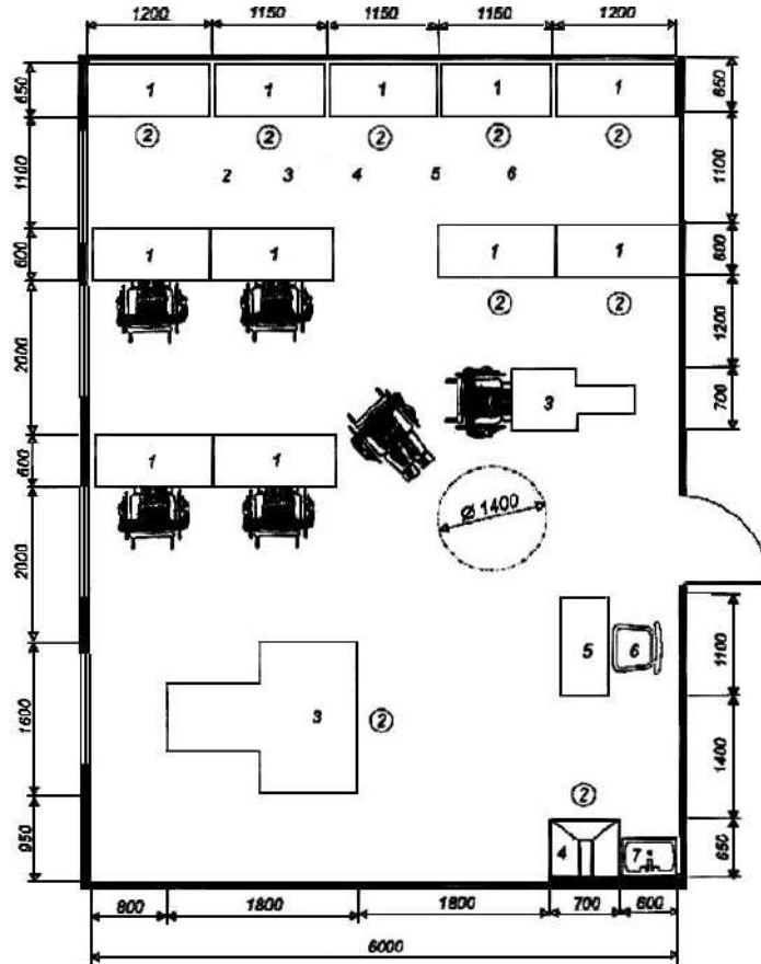
Рис. 11. Пример планировки помещения
