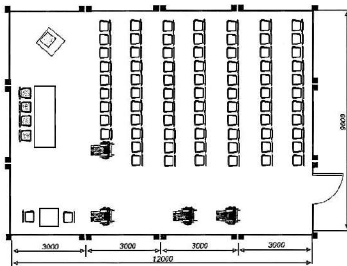
Места инвалидных колясок в помещении для собраний
