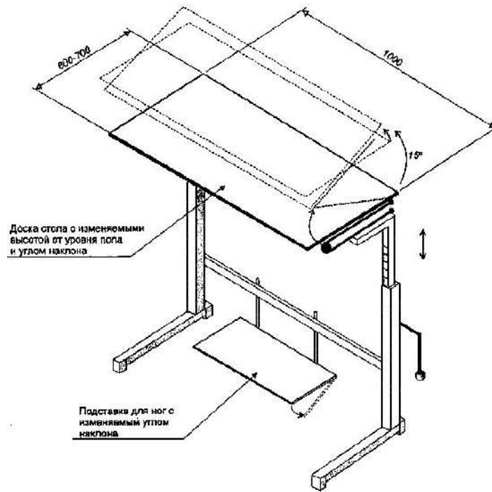
Рис. 12. Трансформируемый рабочий стол для инвалида
