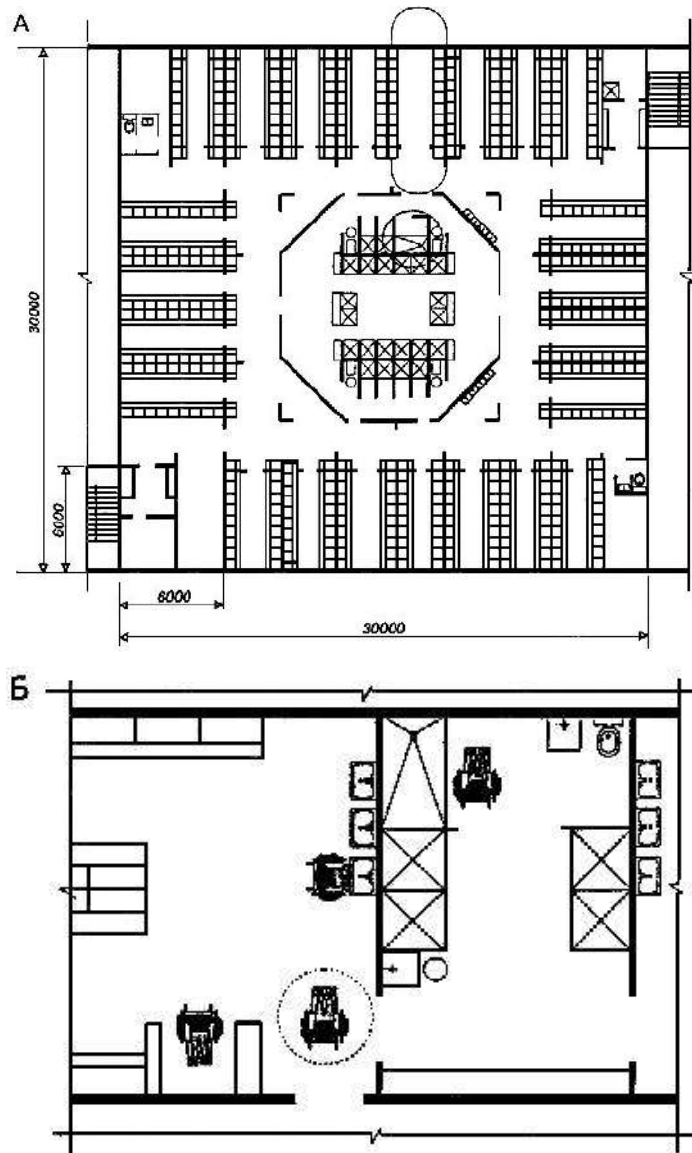
Размещение гардеробной (А) и душевой (Б) для инвалидов в общем гардеробном блоке. Индивидуальная кабина инвалида в общей душевой
