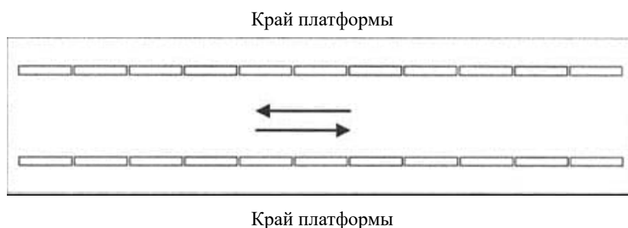
Рисунок А.4 — Форма рифления — одноэлементная тактильная полоса с плоской вершиной (щучиния), используемая для обустройства протяженных предупреждающих ТНУ вдоль края платформ различного назначения
