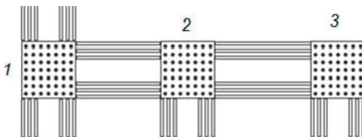
Рисунок А.9 — Применение ТНУ для обустройства тактильно обозначенных путей следования при движении в одном направлении (поворот, примыкание, ответвление)
