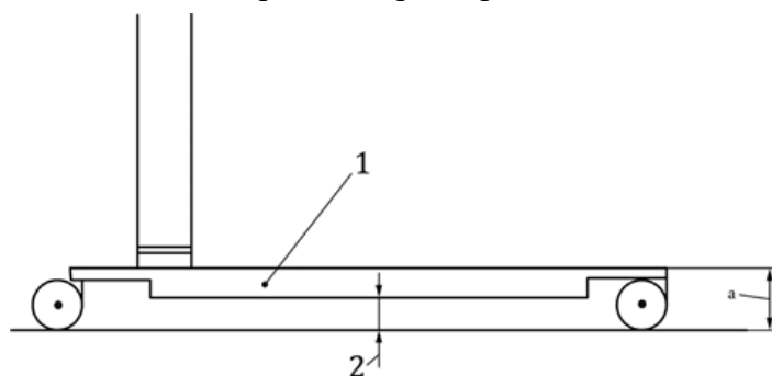
Рисунок 12 — Основные термины и размеры для потолочного подъемника
