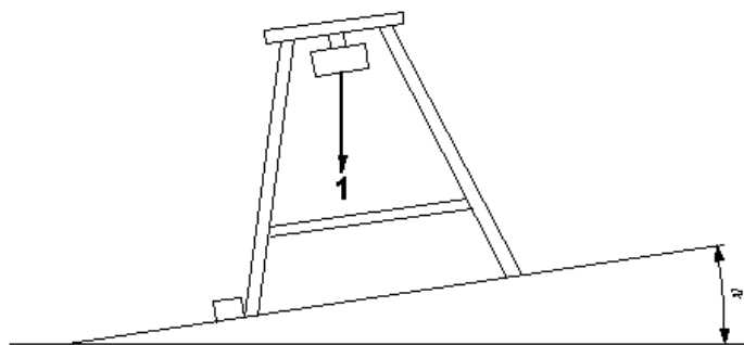
Рисунок 16 — Испытание на устойчивость стационарных автономных подъемников
