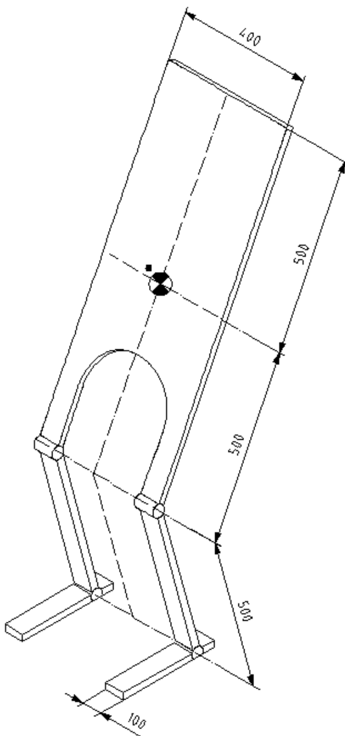
Рисунок 2 — Манекен для испытаний мобильных подъемников для перемещения человека в положении стоя
