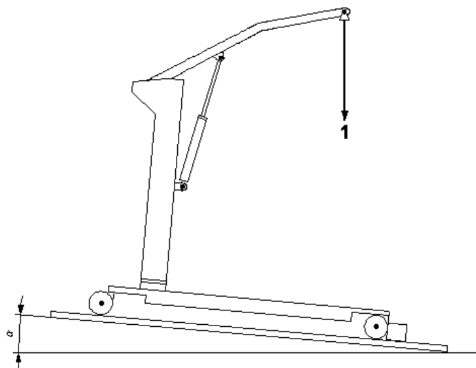
Рисунок 14 — Пример испытания на устойчивость при движении вперед
