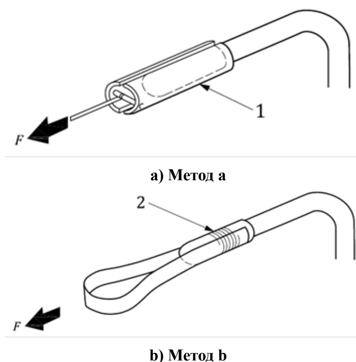
Рисунок 6 — Методы приложения нагрузки к рукоятке
