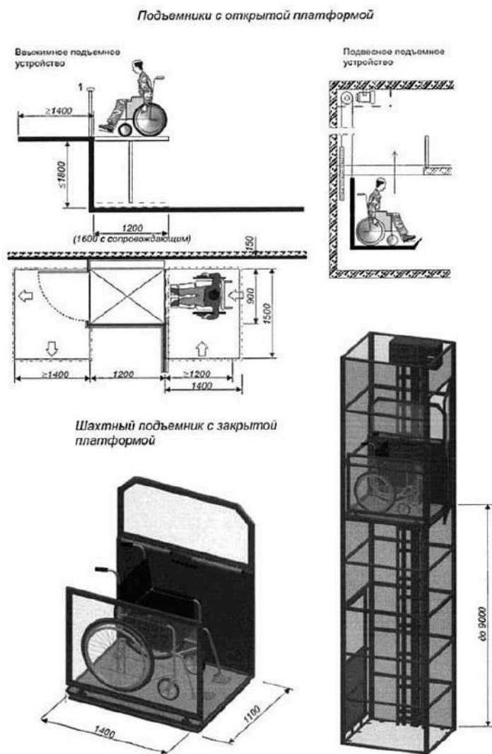
Рисунок В.33 - Параметры вертикальных подъемников
