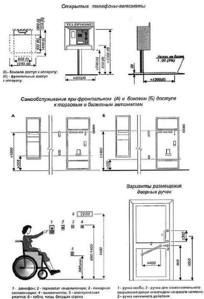
Рисунок Г.6 - Досыгаемость оборудования
