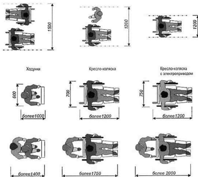
Минимальные габариты полосы движения для детей-инвалидов.
