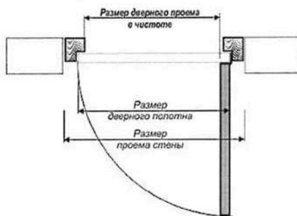
Измерение проемов входных дверей
