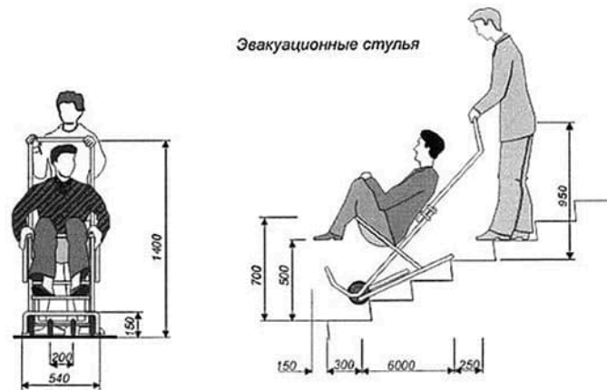
Рисунок В.34 - Автономные транспортные устройства
