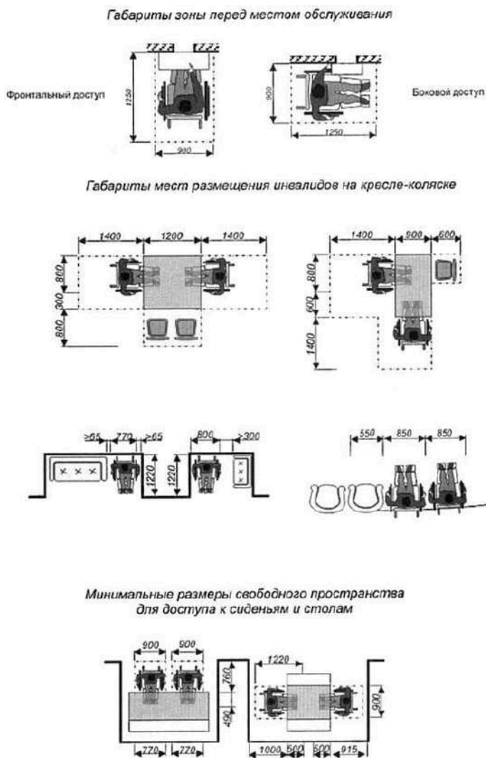
Рисунок Г.5 - Габариты у мест обслуживания
