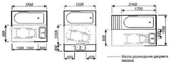
Рисунок Г.9 - Функциональные зоны и примеры оборудования ваннных комнат
