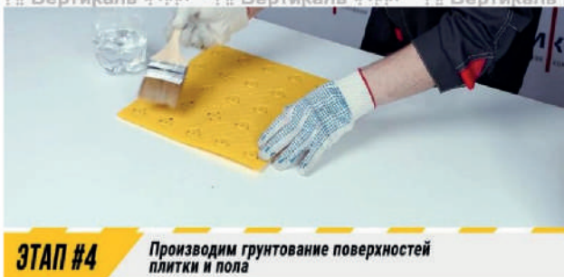
ЭТАП #4 Производим грунтование поверхностей плитки и пола
