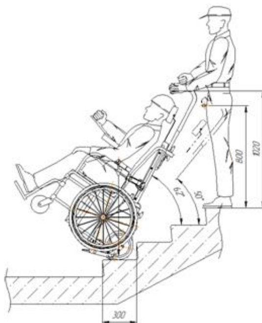
Рис.8. Движение подъёмника по ступеням
